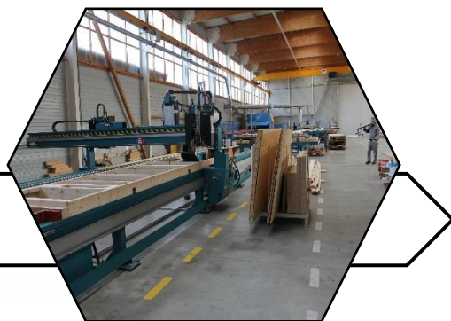
MACH DIFFUSION
